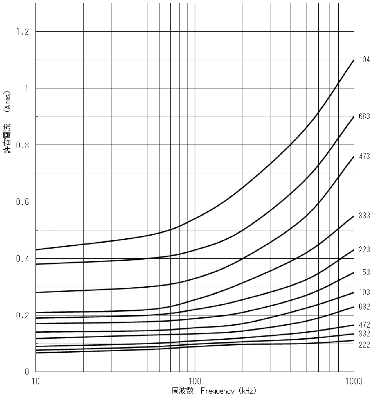
周波数別許容実効電流値 MDD 1250VDC(500VAC)
